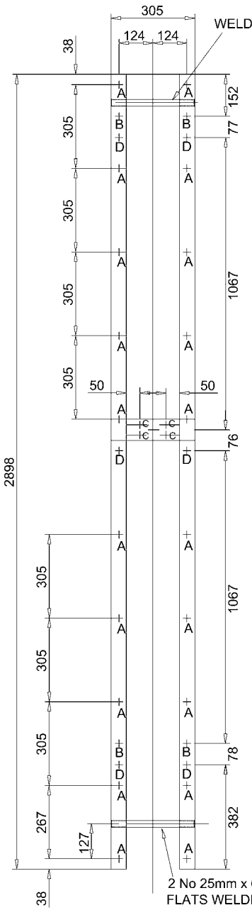
ELEVATION
